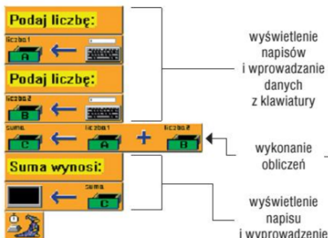
Rys. 2. Program w środowisku Baltie
