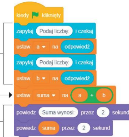
Rys. 3. Program w środowisku Scratch
